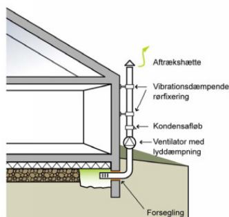
Aktivt radonsug med ekstern rørledning og ventilator. Brønden er udført ved at bore gennem fundamentet og grave ud til en brønden under gulvkonstruktionen.
