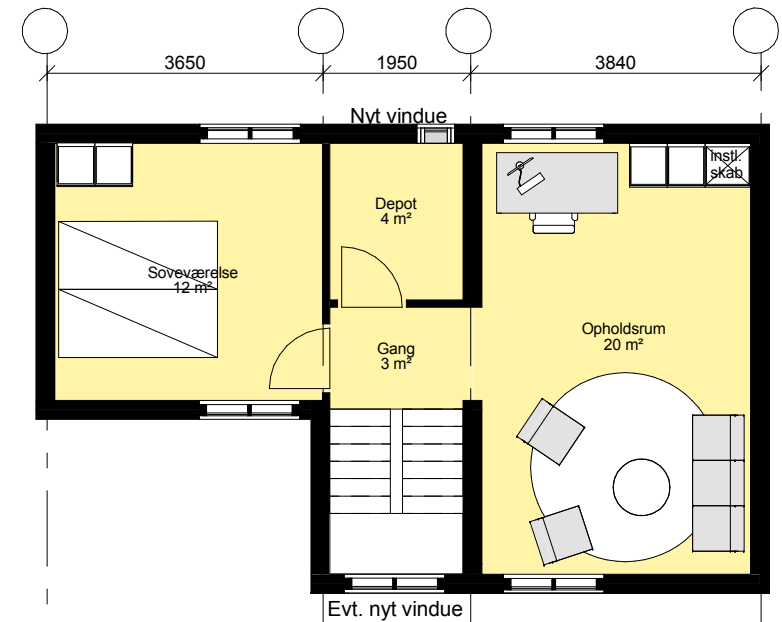
2. salsplan type 2 Sammenlægning af B3+A2 M 1:100
