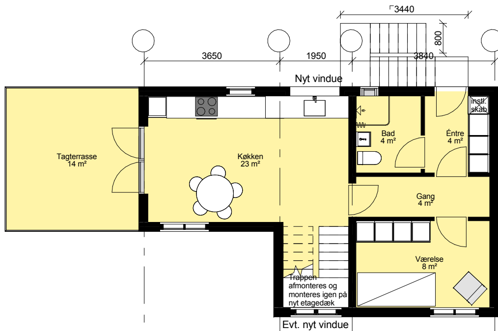
1. salsplan type 2 Sammenlægning af B3+A2 M 1:100
